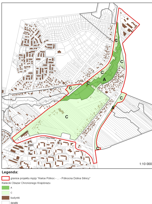
Rys. 12. Kielecki Obszar Chronionego Krajobrazu z podziałem na strefy krajobrazowe.
