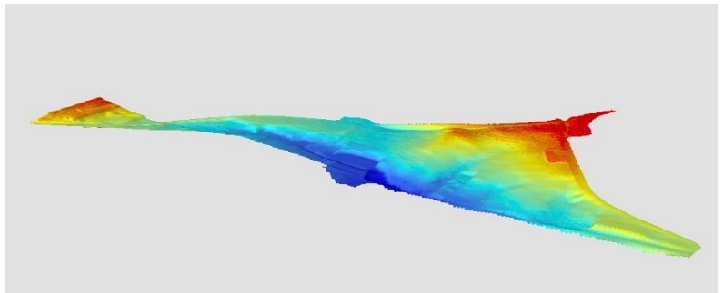
Rys. 2. Rzeźba terenu opracowania (widok od strony zachodniej).
