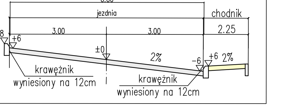
SCHEMAT PRZKROJU DROGI km 0+540 - koniec opracowania
