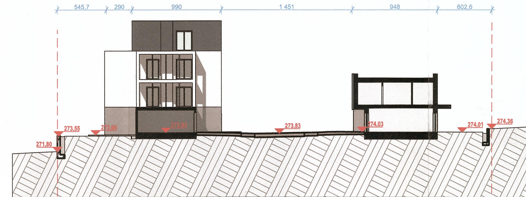
PRZEKRÓJ A-A
