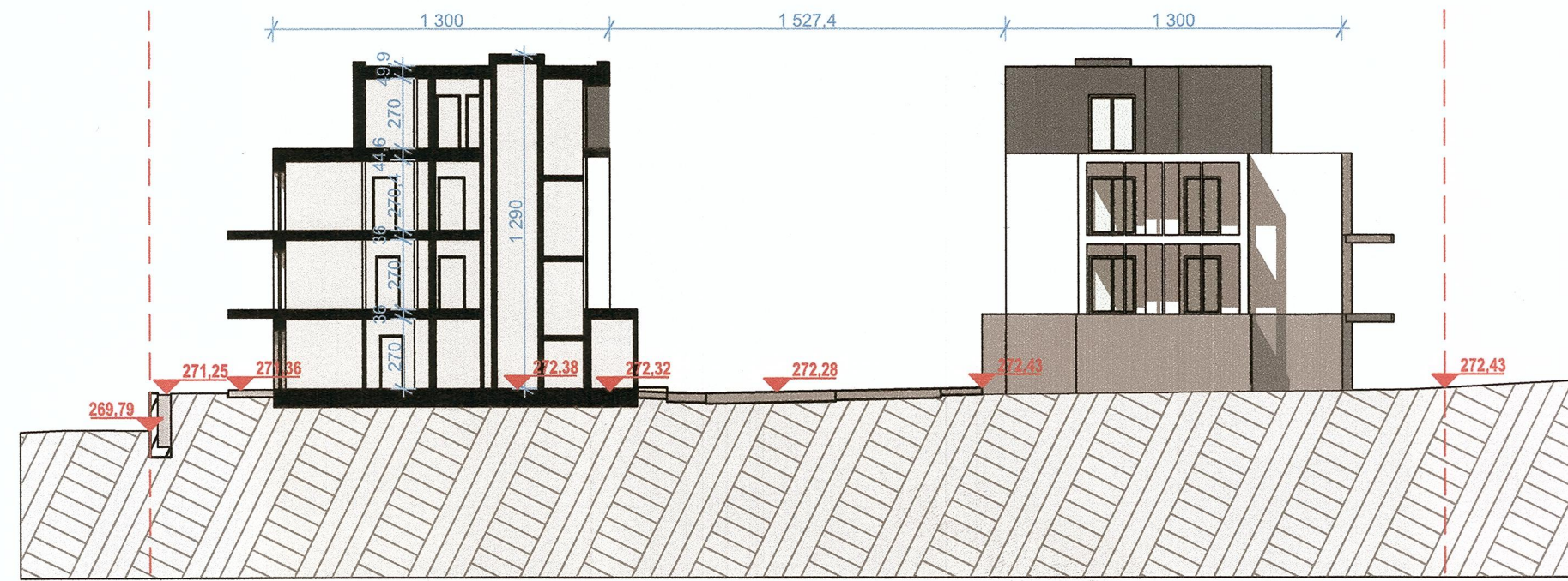
PRZEKRÓJ B-B
