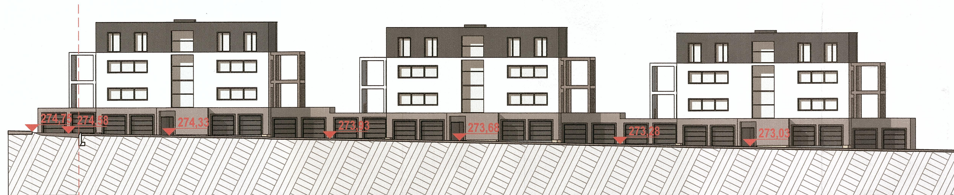
ELEVACJA D-D
