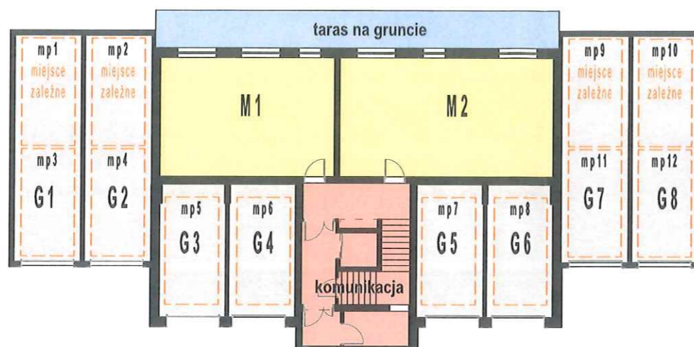
RZUT PARTERU
